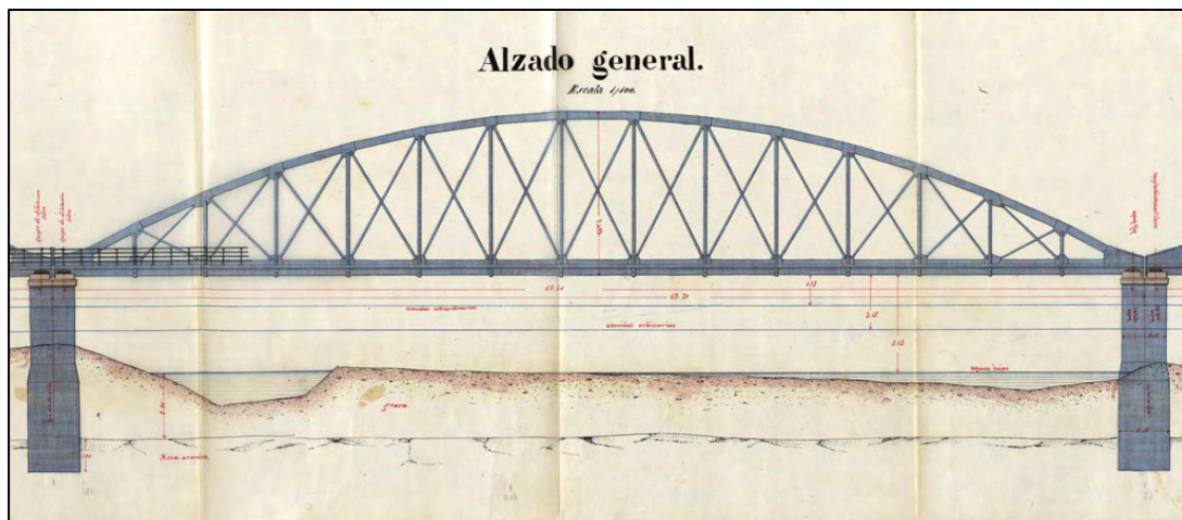
Proyecto de puente de hierro sobre el río Cinca en Monzón. 1876
